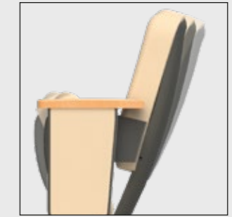
El espaldar puede inclinarse en tres posiciones, de 15°, 18° y 21°. El asiento puede abatirse a 90° en SSE, y a 75° en la versión estándar.
